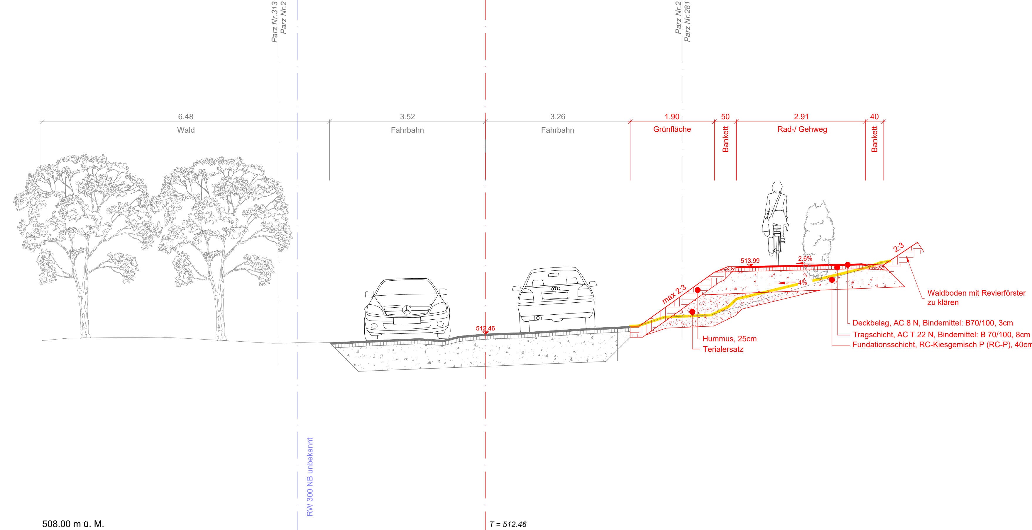
Normalprofil Radweg abgesetzt Hermrigen 1360.00
