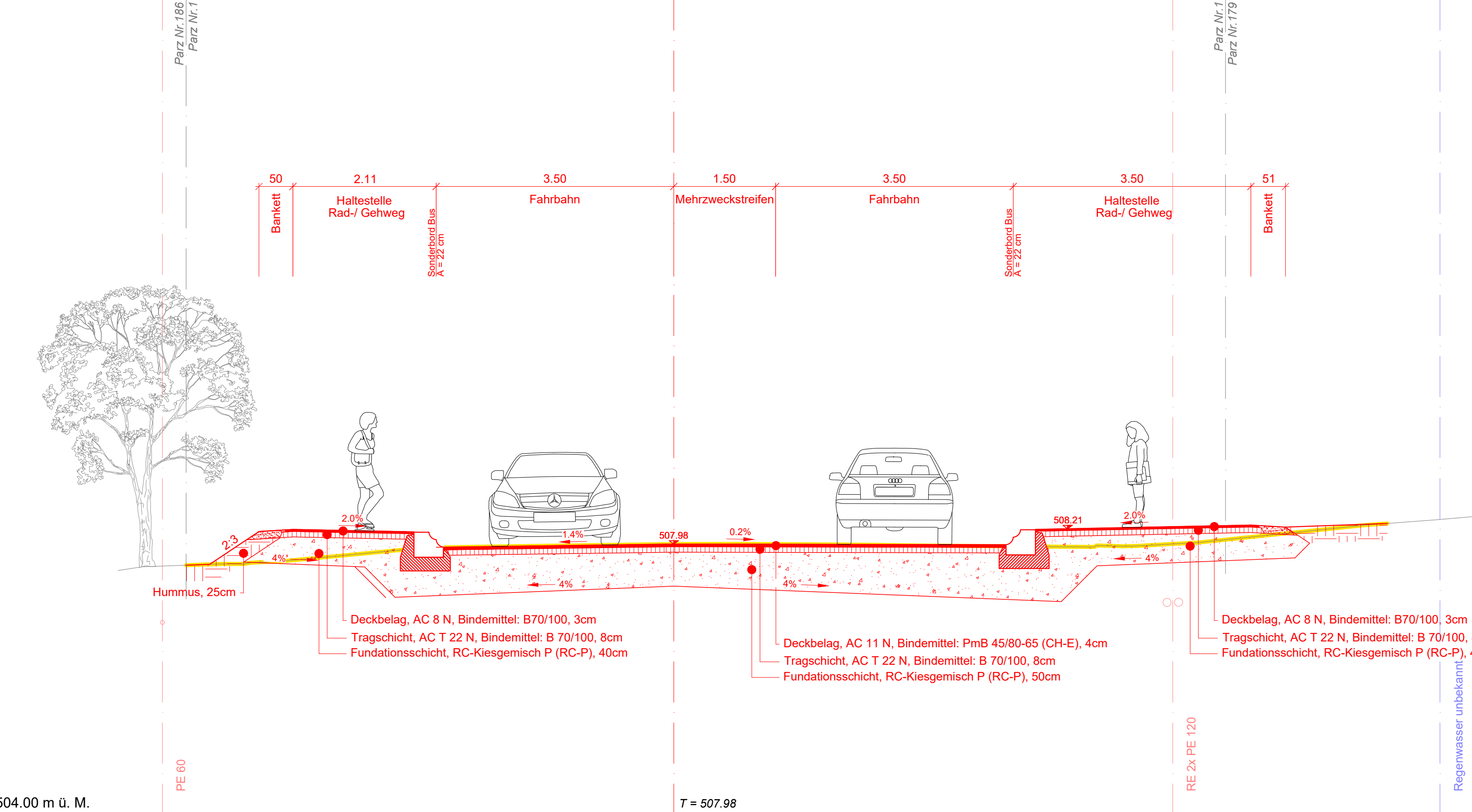
Normalprofil Haltestelle Friedhof 1460.00
