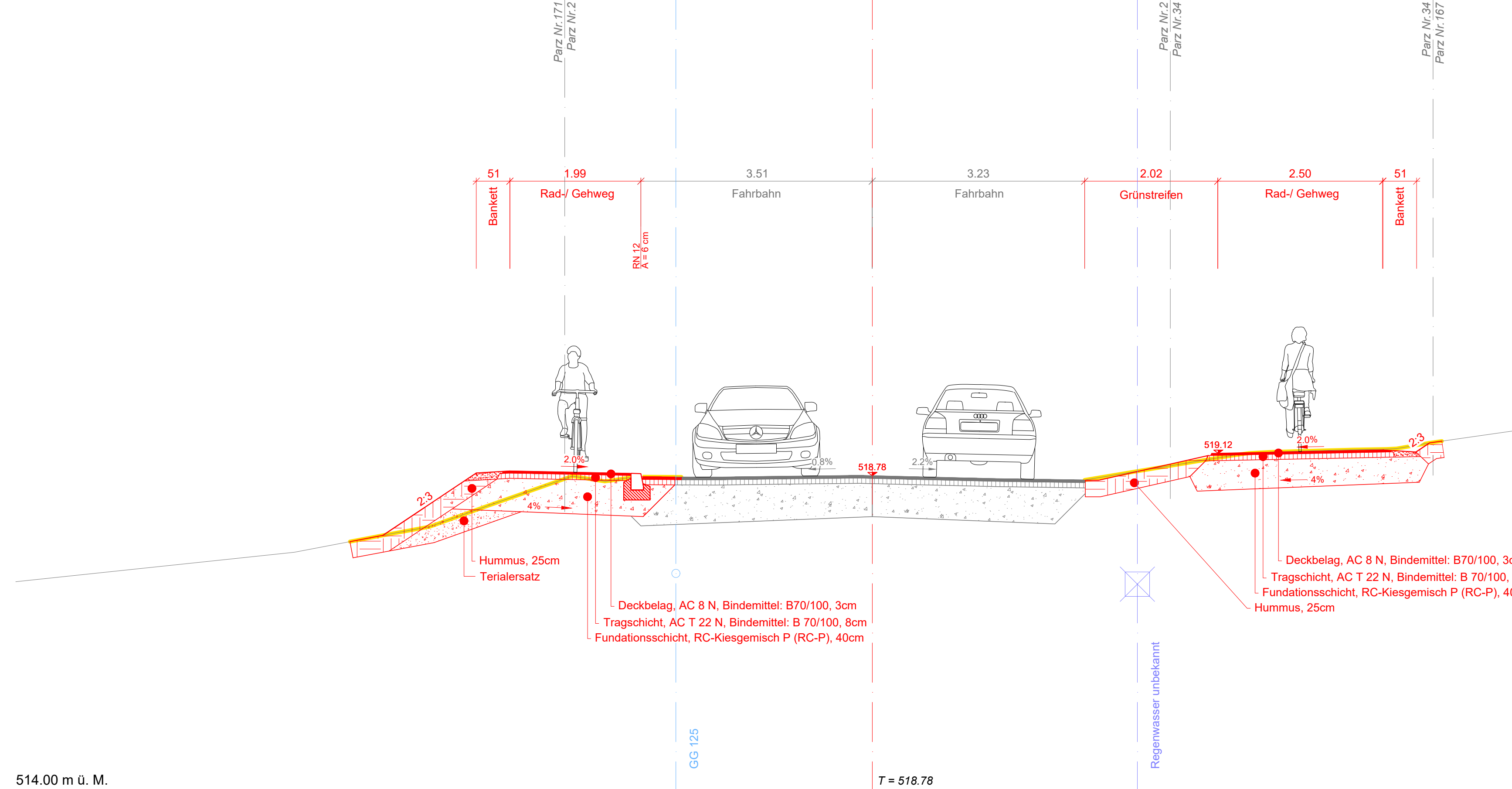
Normalprofil Radweg beidseitig 1070.00
