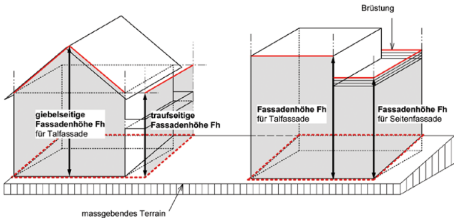
Figur 4.2.a Fassadenhöhe
