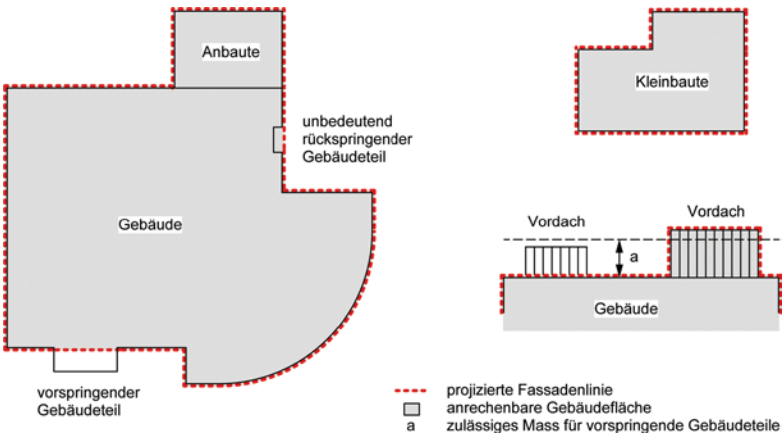
Figur 7.4 Anrechenbare Gebäudefläche
