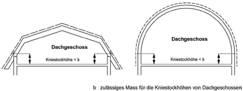
Figur 5.3 Dachgeschosse
